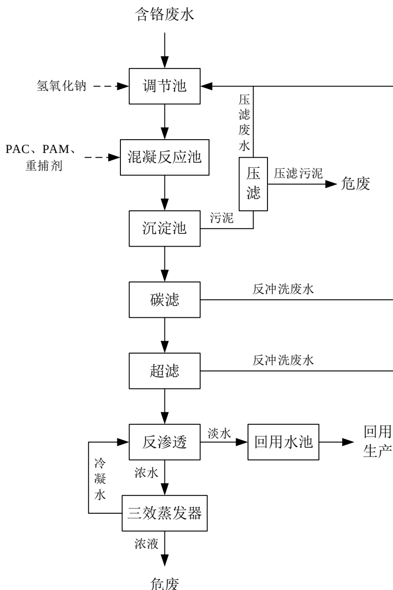
图 3-11 含铬废水处理工艺流程图
