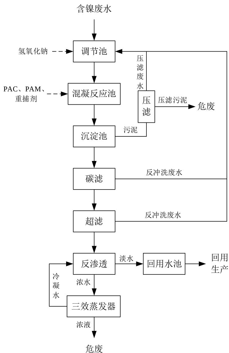
图 3-10 含镍废水处理工艺流程图
