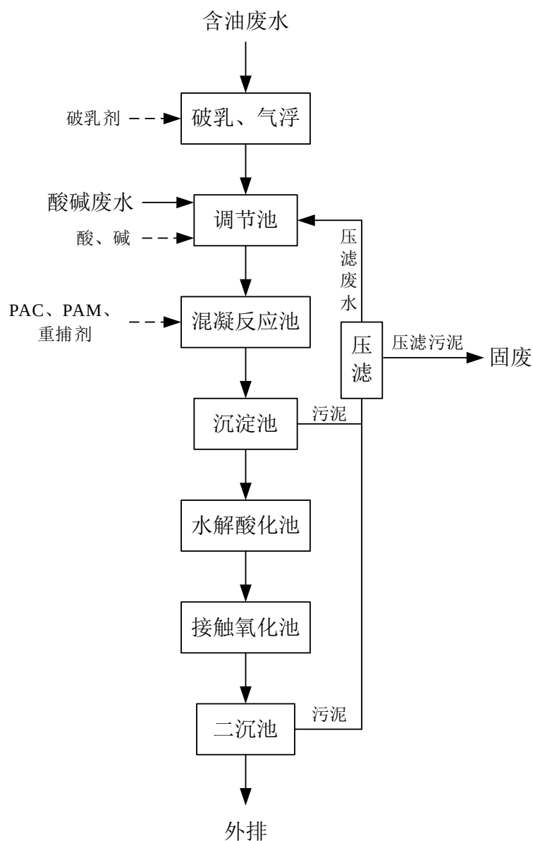
图 3-13 镀前综合废水处理工艺流程图
