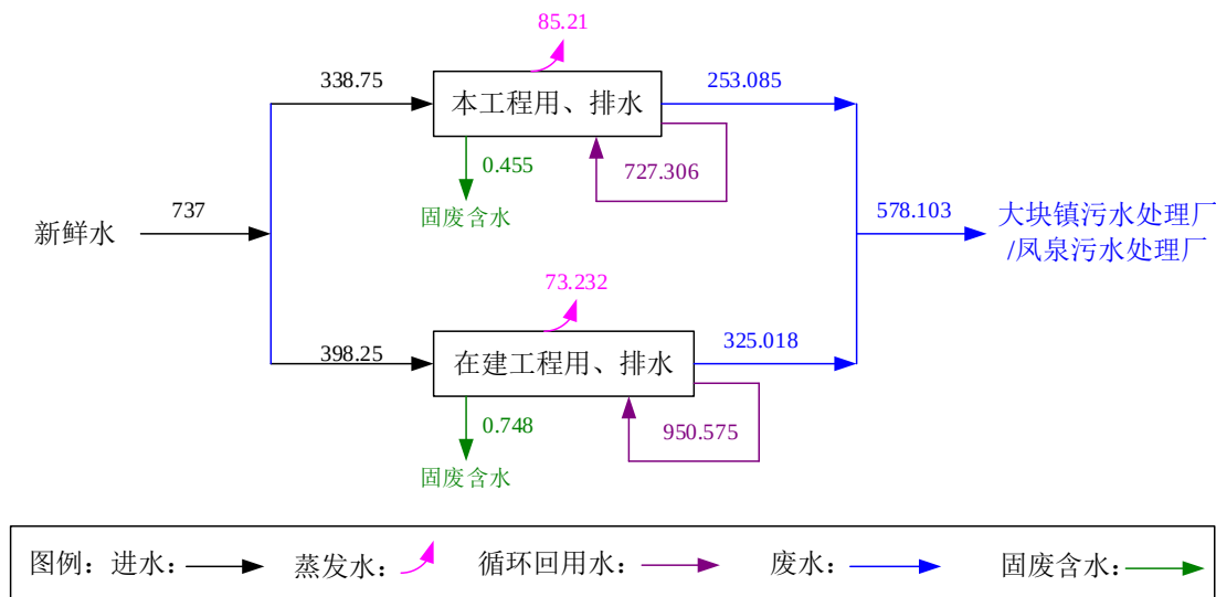
图 3-9 全厂水平衡图 单位：m³/d
