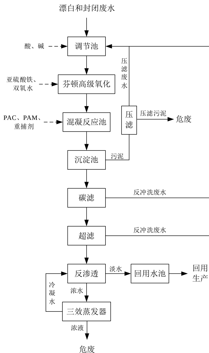
图 7-3 漂白和封闭废水处理工艺流程图
