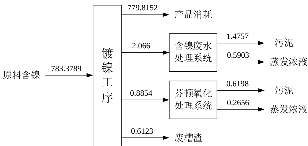
图 3-6 电池钢壳镍平衡图 单位: t/a
