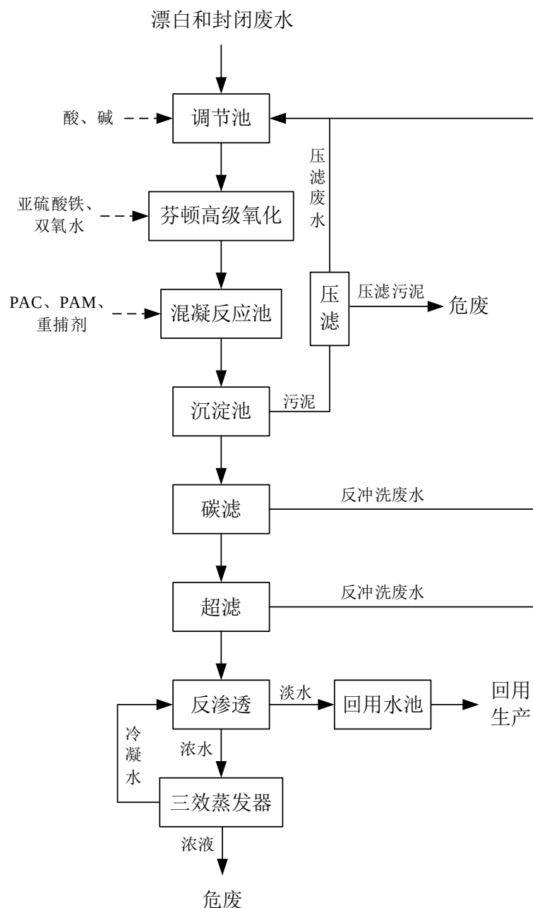
图 3-12 漂白和封闭废水处理工艺流程图
