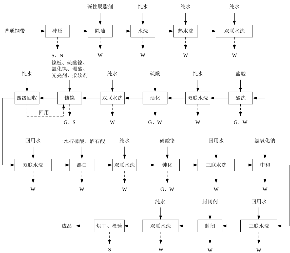
图 3-5 电池钢壳工艺流程及产污环节图
