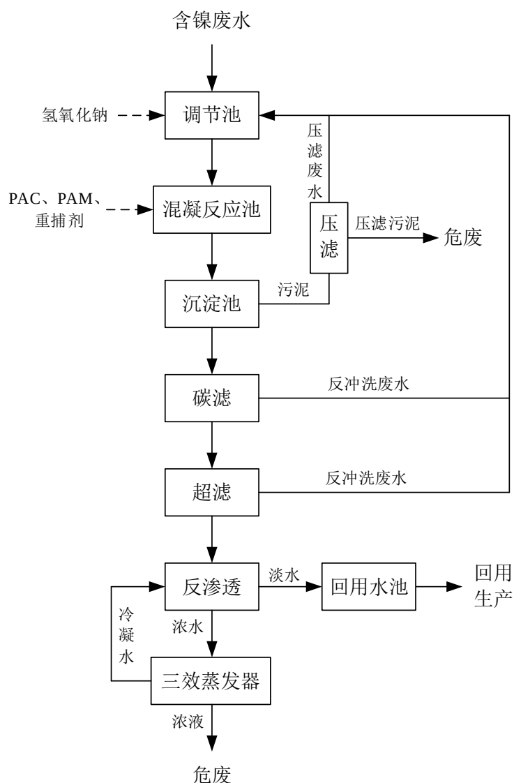
图 7-1 含镍废水处理工艺流程图
