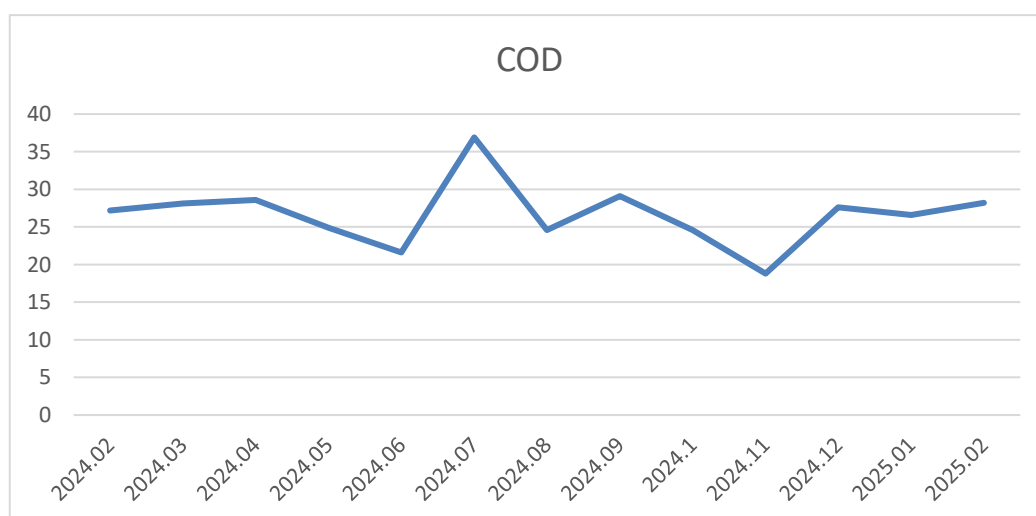
图 4-6 民生渠入共渠口断面近期水质 COD 浓度折线图
