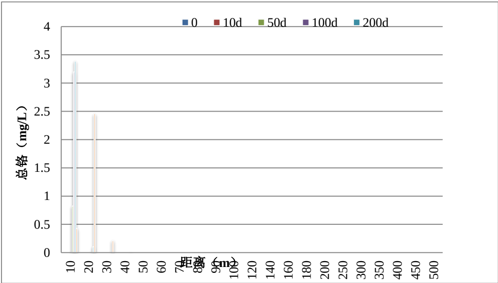
图 5-16 总铬影响范围示意图
