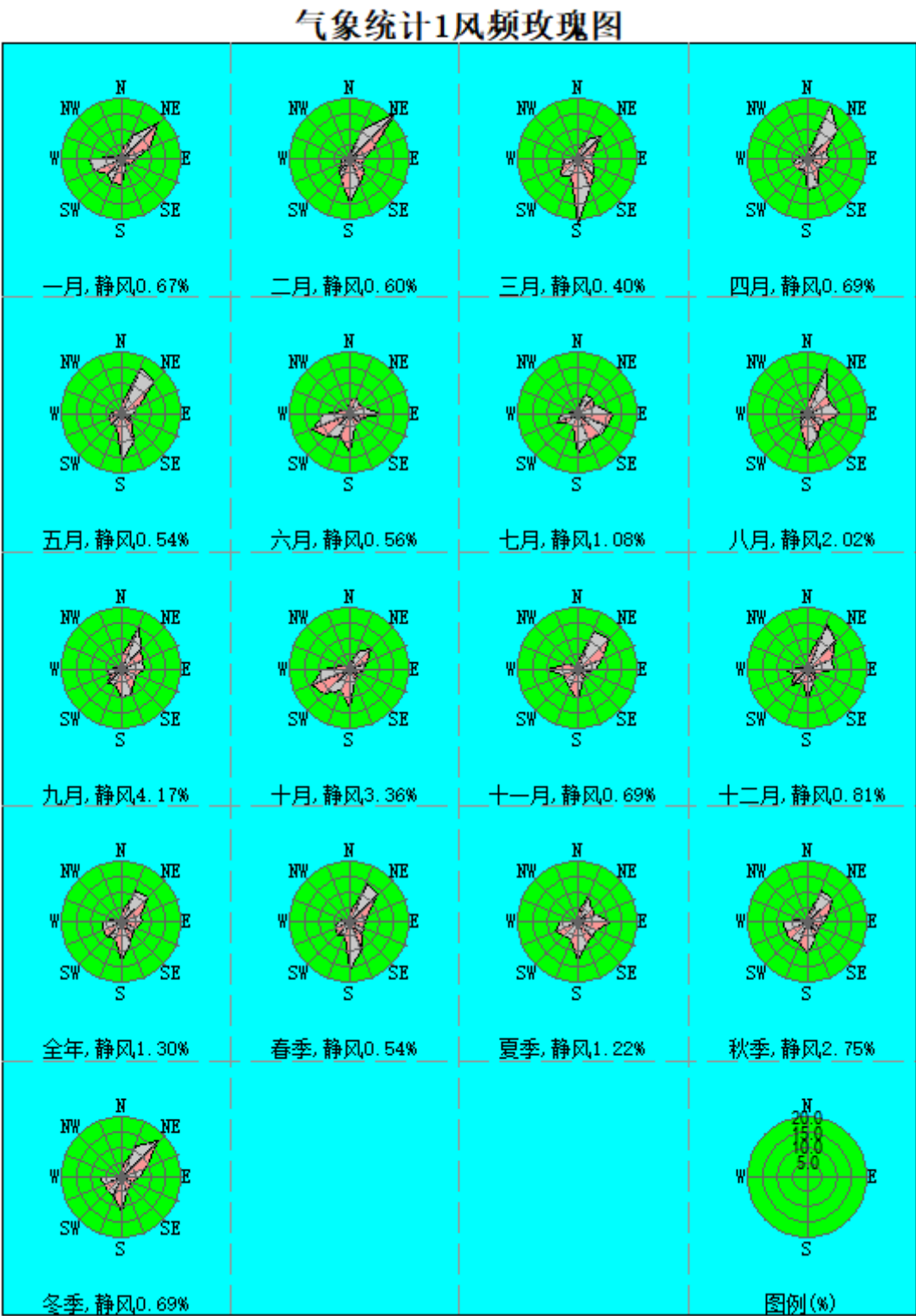
图 5-11 全年及各季风向频率
