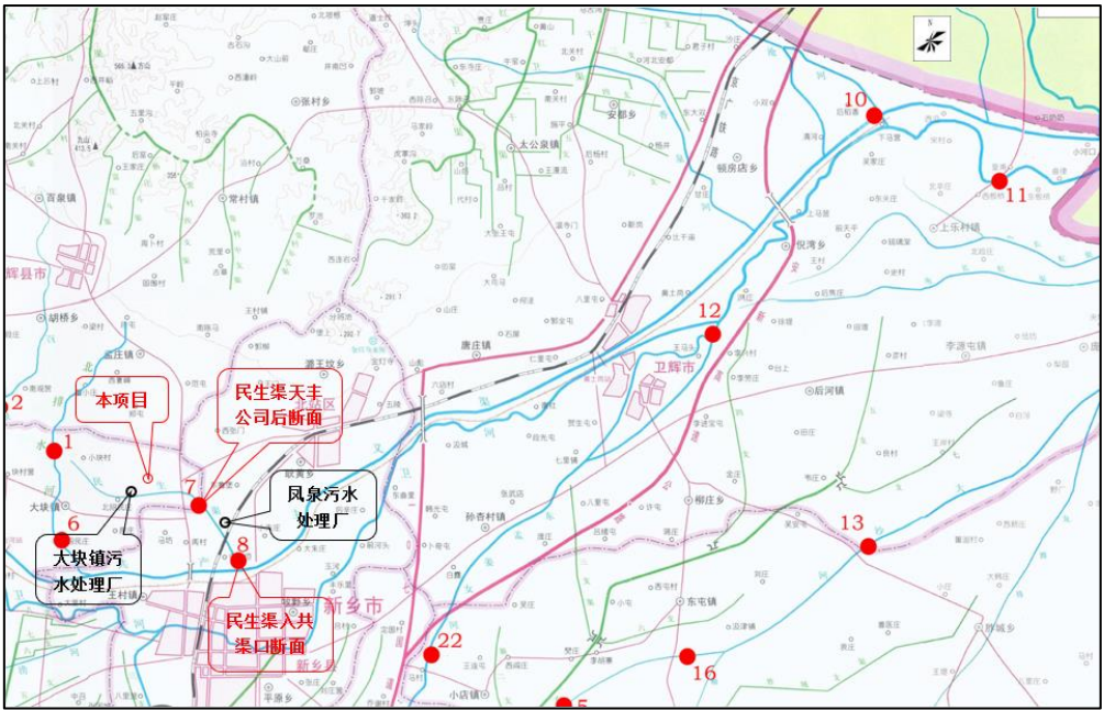
图 4-2 项目附近地表水体分布示意图
