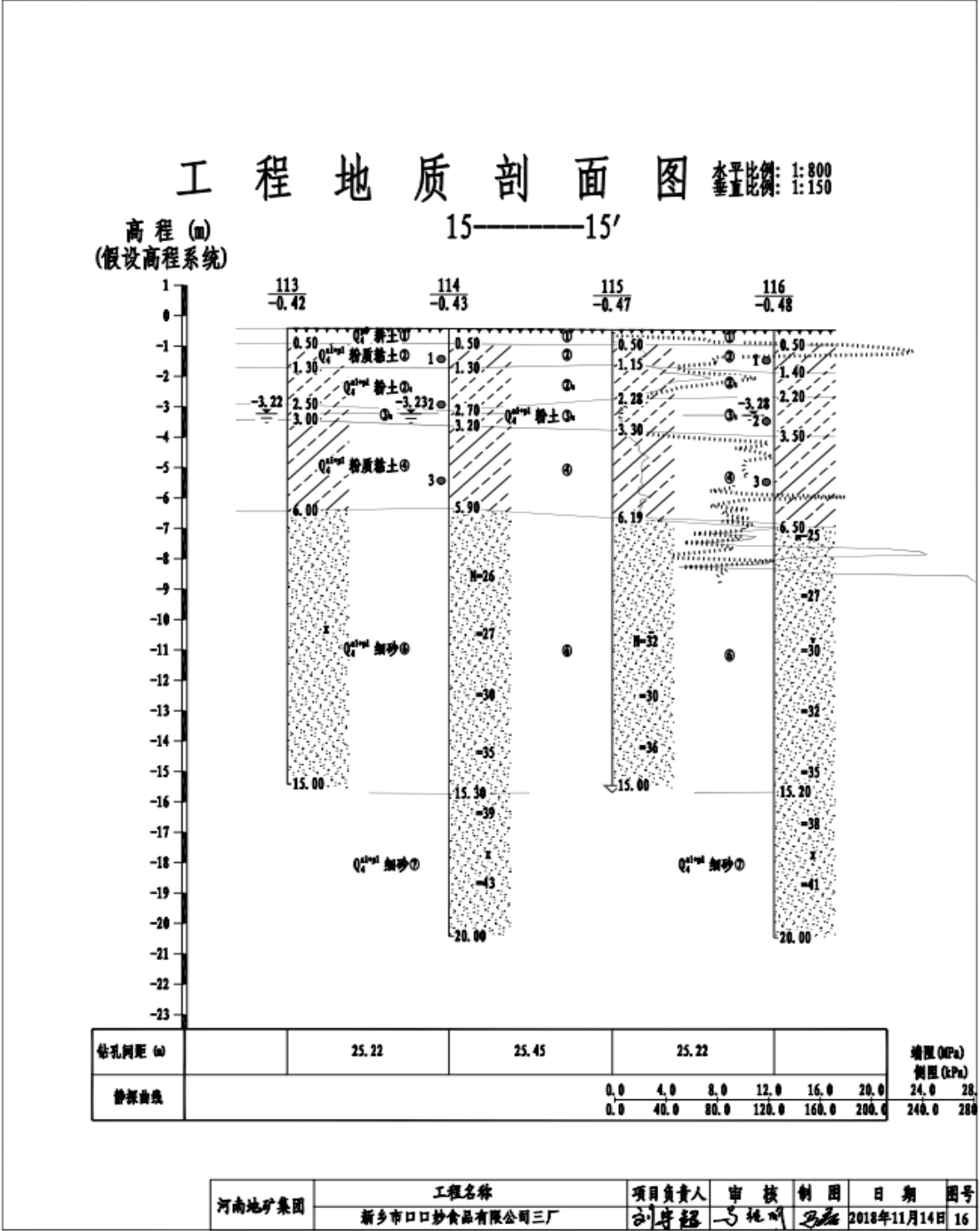
图 5-12 工程地质剖面图
