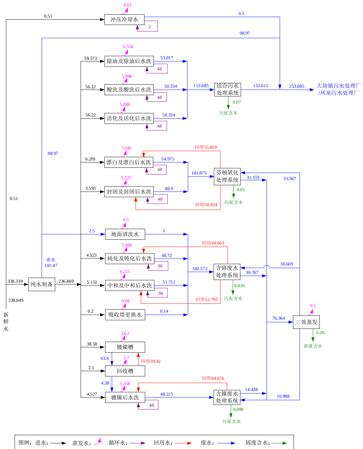
图 3-8 本工程水平衡图 单位：m³/d
