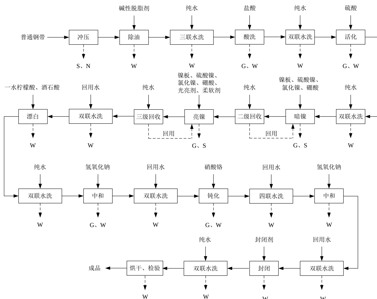
图 3-2 负极底盖工艺流程及产污环节图
