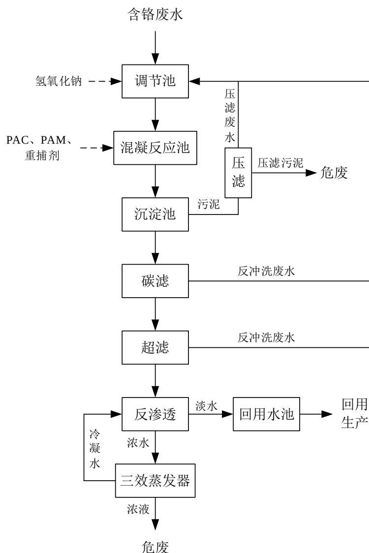
图 7-2 含铬废水处理工艺流程图
