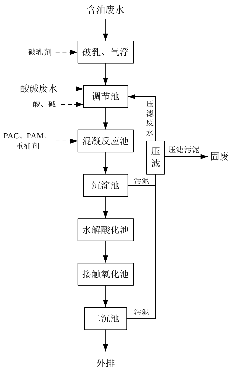
图 7-4 镀前综合废水处理工艺流程图
