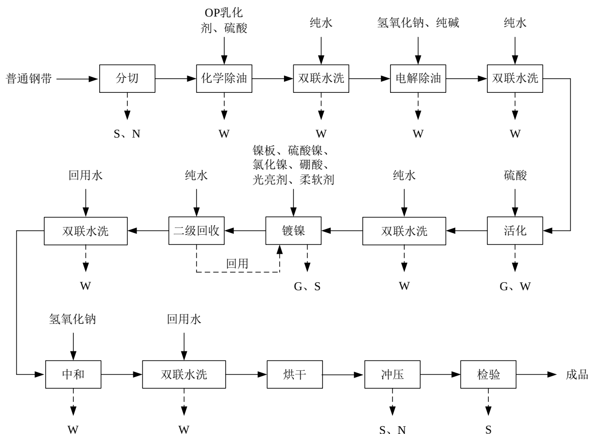
图 3-3 电池连接件工艺流程及产污环节图
