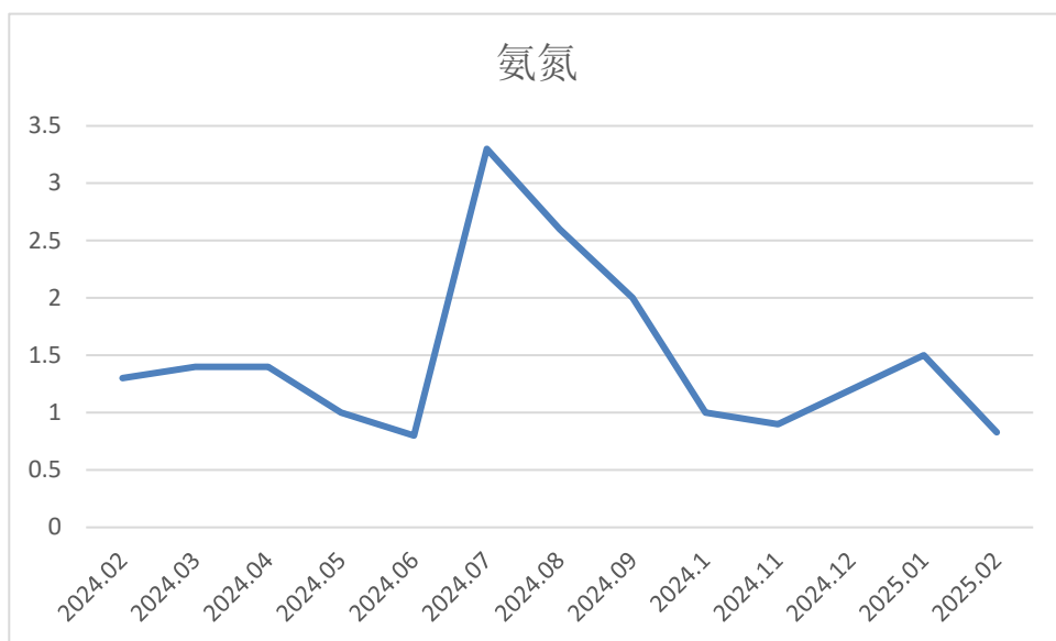
图 4-7 民生渠入共渠口断面近期水质 \text{NH}_3\text{-N} 浓度折线图
