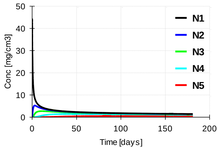
图 5-20 本项目土壤石油烃的预测结果图
