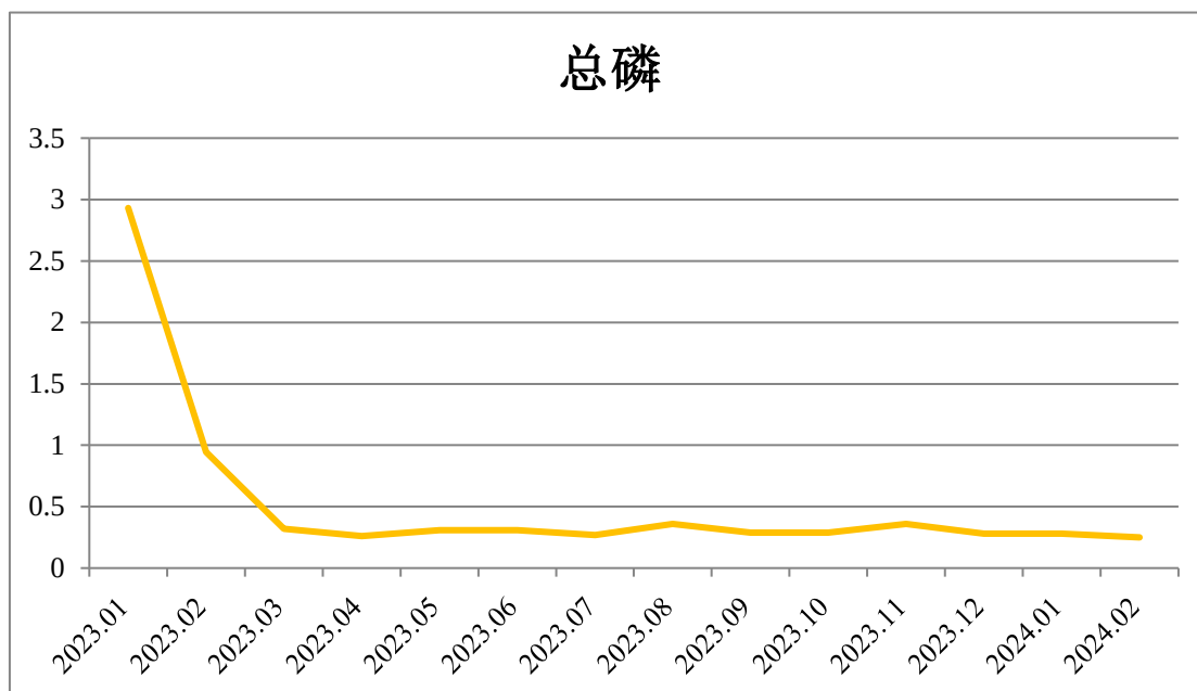
图 4-5 民生渠天丰公司后断面近期水质 TP 浓度折线图
