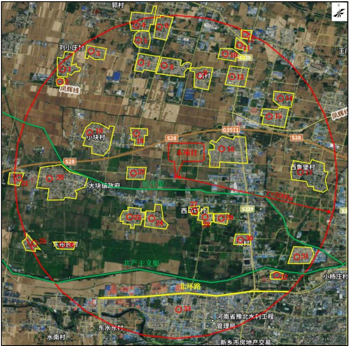
图 6-2 本项目周围环境敏感点示意图
