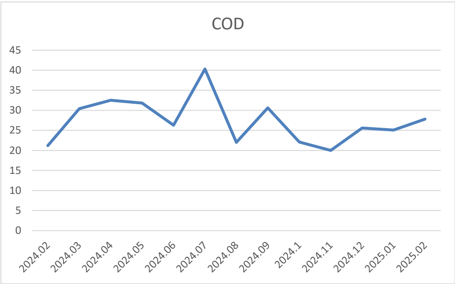
图 4-3 民生渠天丰公司后断面近期水质 COD 浓度折线图
