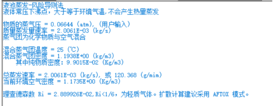
图 6-4 本项目盐酸预测结果
