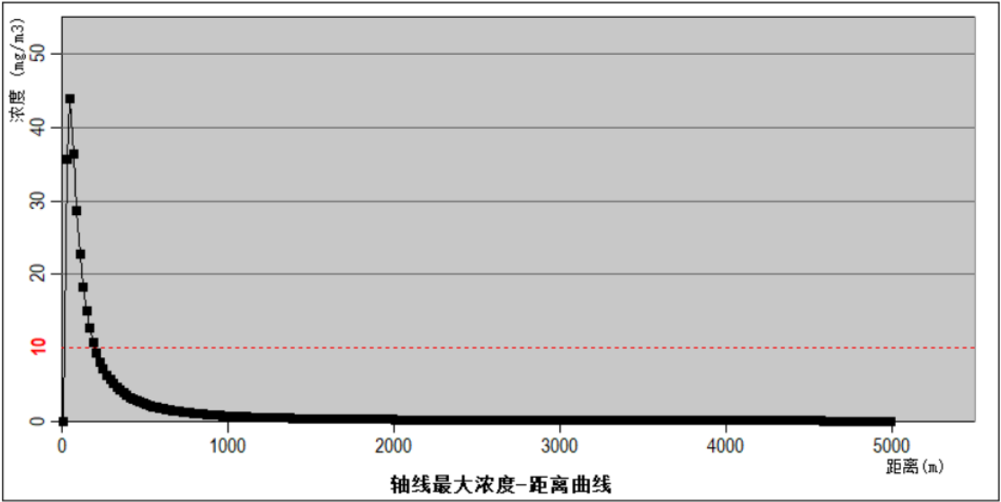
图 6-6 下风向氯化氢最大浓度-距离曲线
