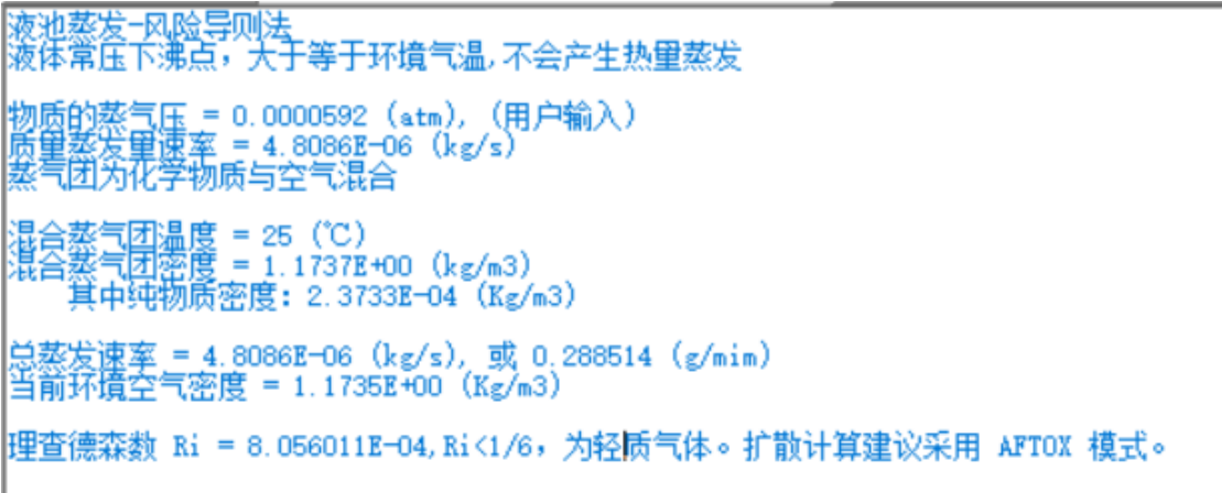
图 6-4 本项目盐酸预测结果
