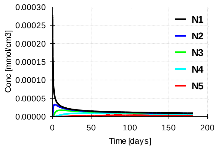
图 5-18 本项目土壤总铬的预测结果图
