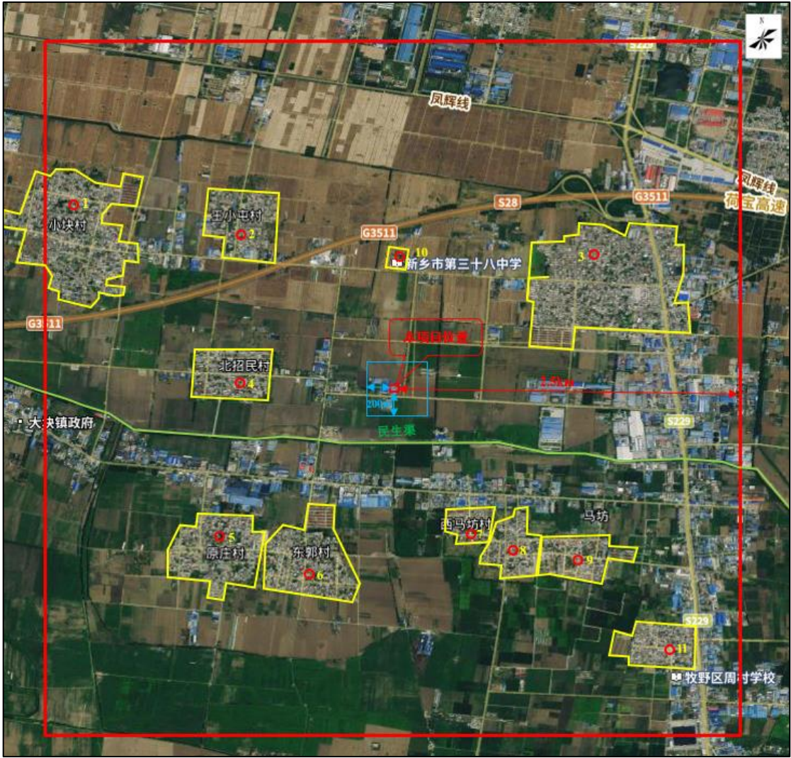
图 2-1 本项目周围环境敏感点示意图
