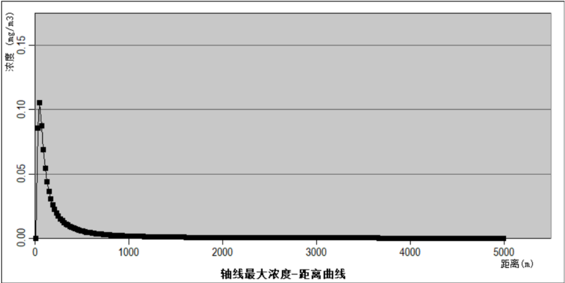
图 6-7 下风向硫酸最大浓度-距离曲线
