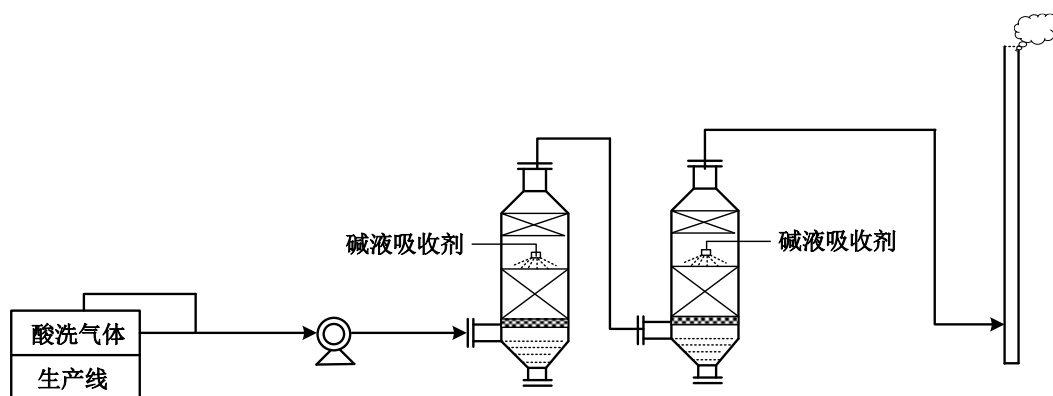
图 7-5 工程含酸废气治理工艺示意图
