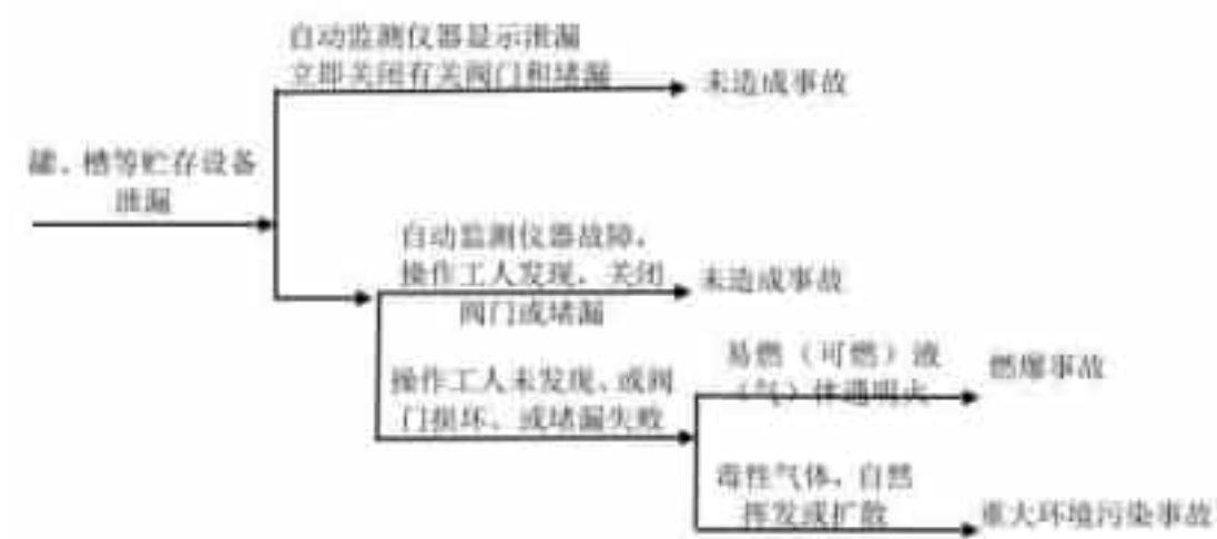
图 6.2-4 储罐系统事件树示意图
