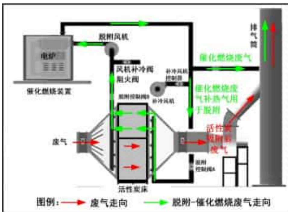
图 3.5-2 活性炭吸附/脱附-催化燃烧装置废气走向图
