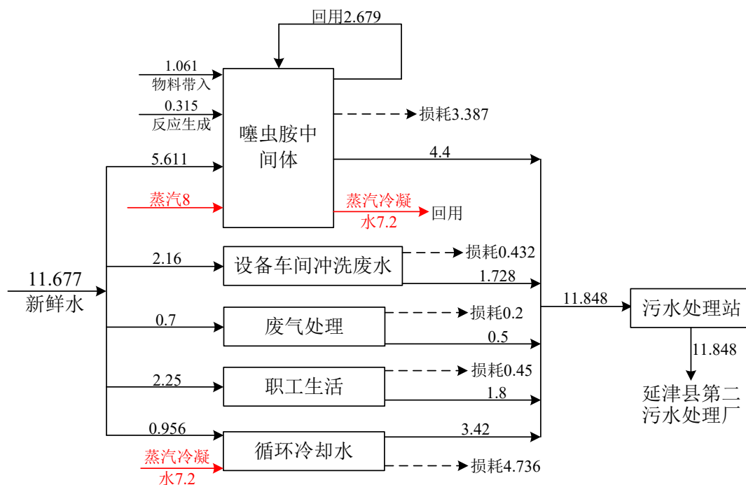
图 3.2-4 “以新带老”后现有工程水平衡示意图
