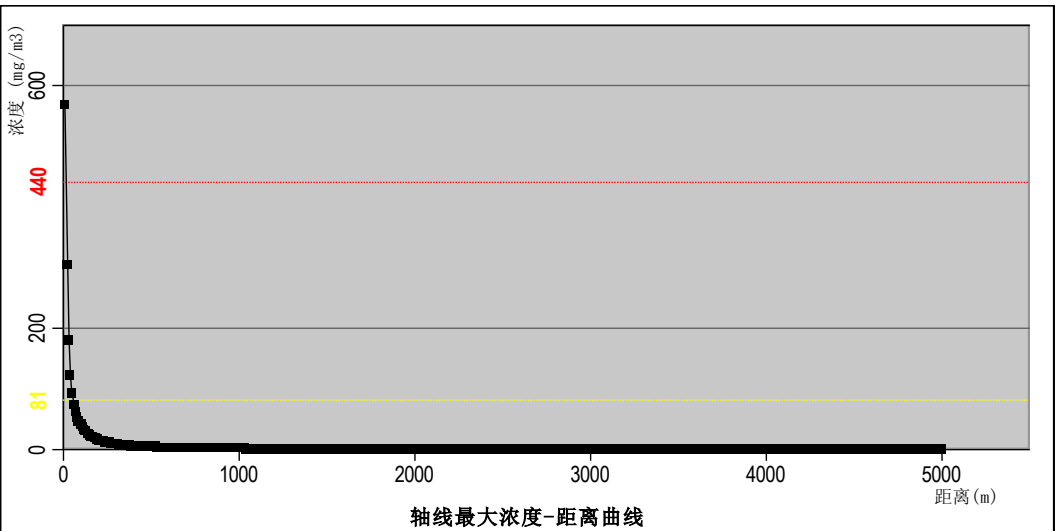
图 6.2-12 最不利气象下风向一甲胺最大浓度-距离曲线
