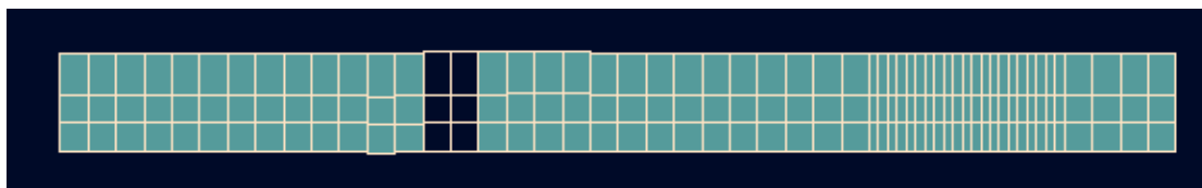
图 5.6-12 模拟区 C-D 剖面垂向剖分图
