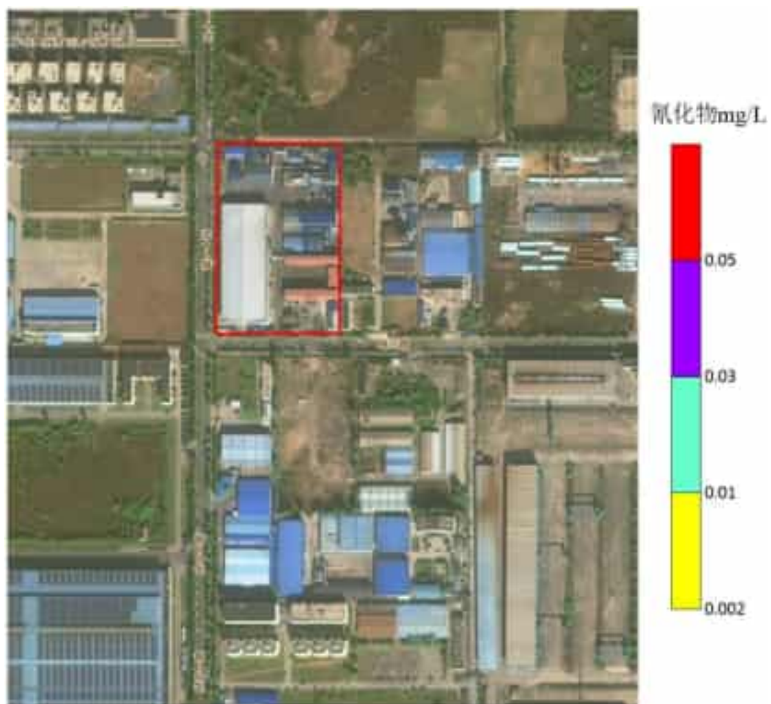
图 5.6-25 3650 天污染晕运移分布图
