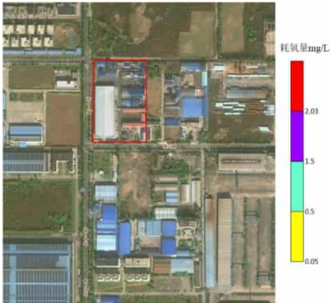
图 5.6-17 3650 天污染晕运移分布图
