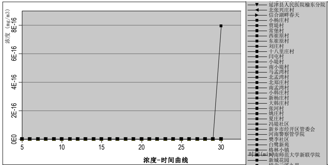
图 6.2-20 最不利气象敏感点一甲胺浓度-时间曲线
