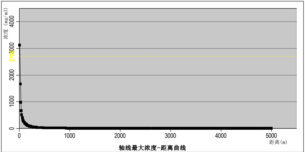
图 6.2-11 最不利气象下风向甲醇最大浓度-距离曲线
