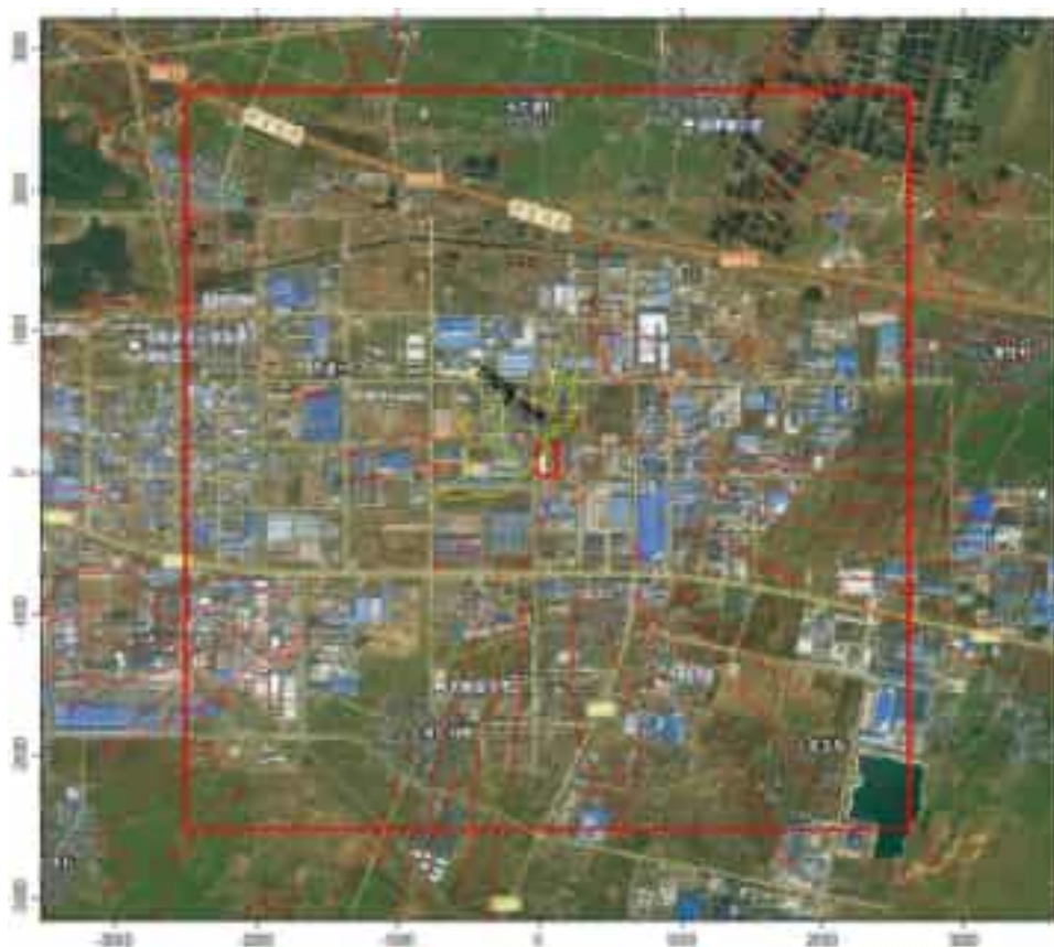
图 5.2-46 一甲胺小时浓度等值线图
