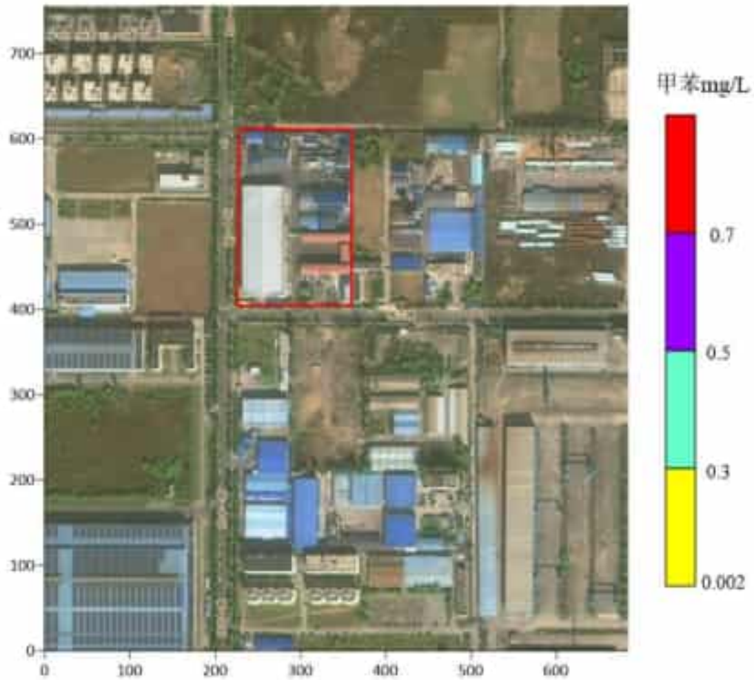
图 5.6-30 7300 天污染晕运移分布图
