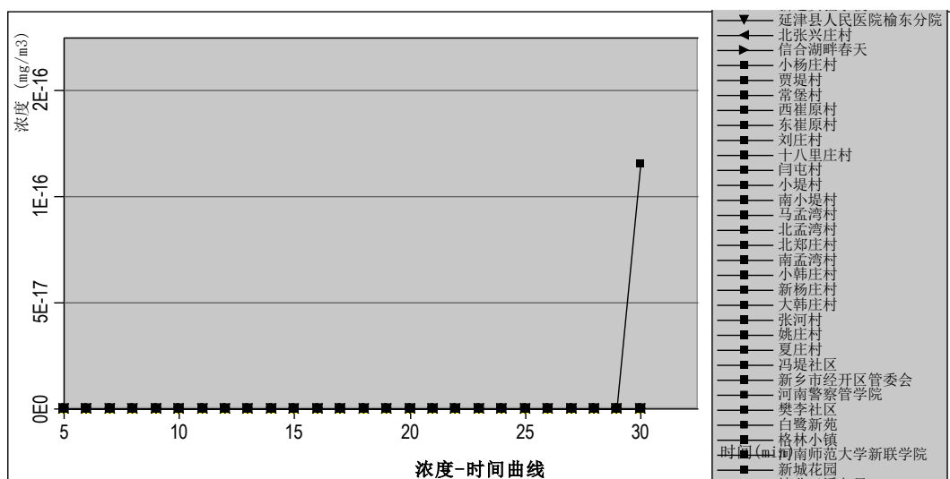
图 6.2-14 最不利气象敏感点乙腈浓度-时间曲线
