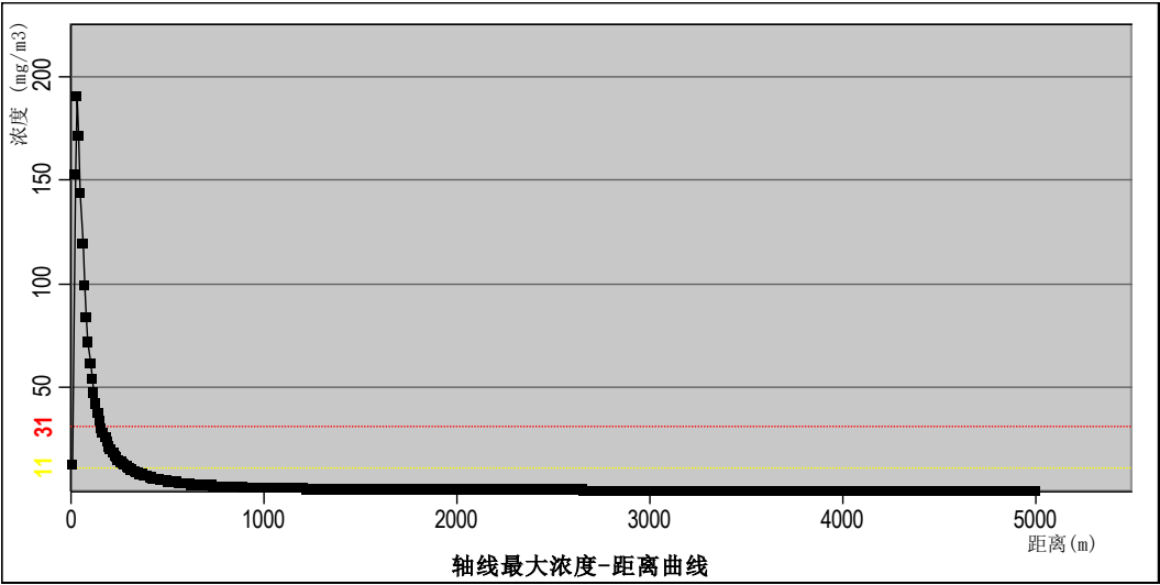
图 6.2-7 最不利气象下风向三氯化磷最大浓度-距离曲线
