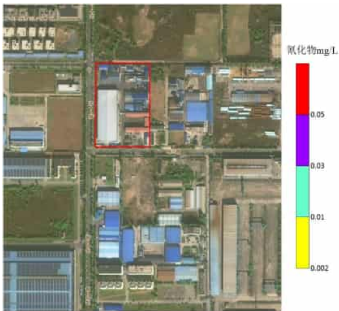
图 5.6-26 7300 天污染晕运移分布图
