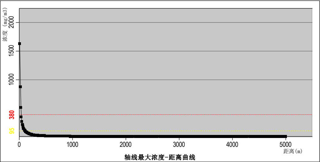
图 6.2-27 最不利气象下风向 CO 最大浓度-距离曲线
