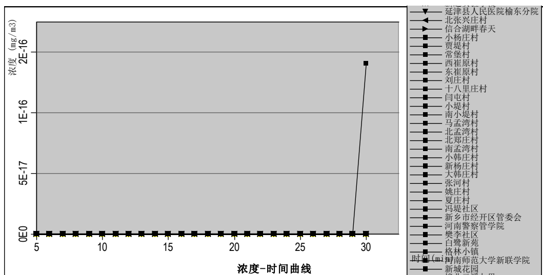
图 6.2-15 最不利气象敏感点三氯化磷浓度-时间曲线
