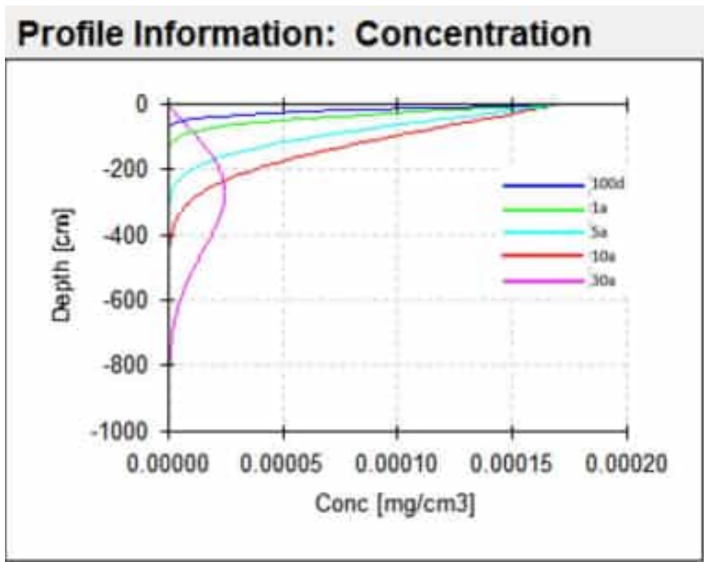
图 5.7-3 土壤甲苯在不同水平年沿土壤迁移情况图
