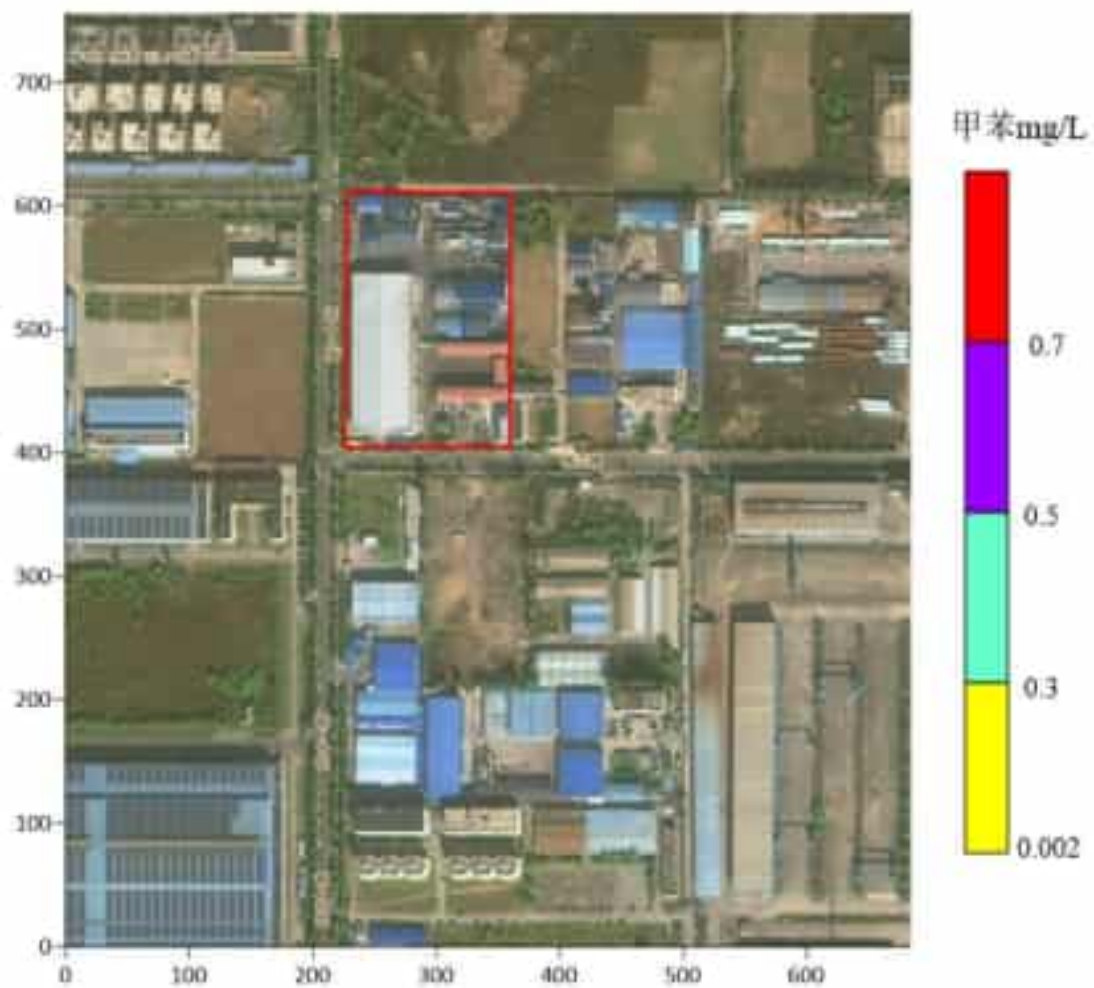
图 5.6-29 3650 天污染晕运移分布图
