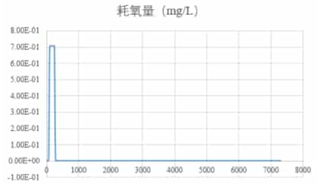
图 5.6-31 厂区下游边界地下水耗氧量污染趋势图
