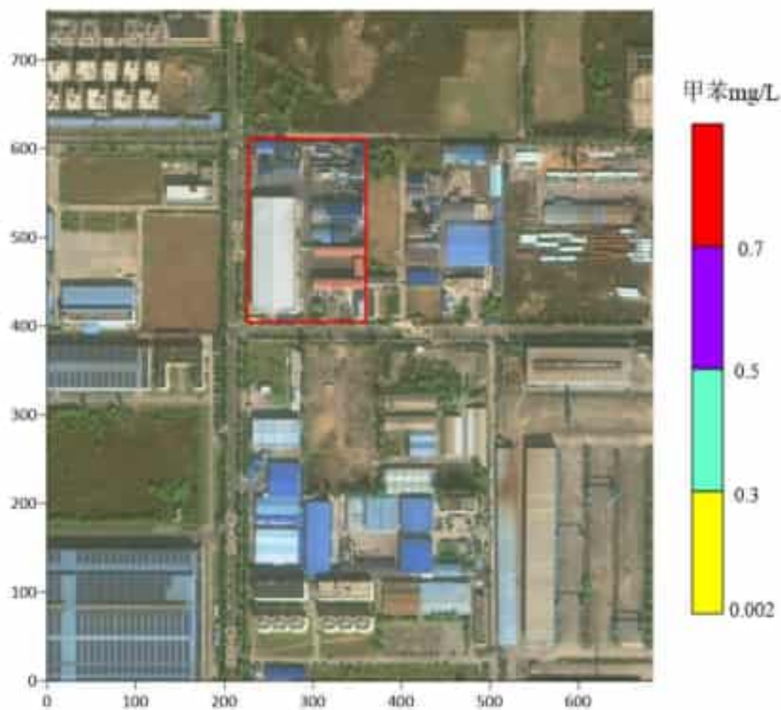
图 5.6-27 100 天污染晕运移分布图
