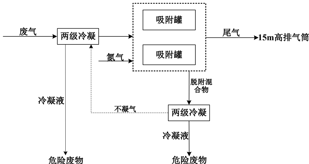
图 3.5-1 两级冷凝+活性炭吸附/脱附装置工艺流程图
