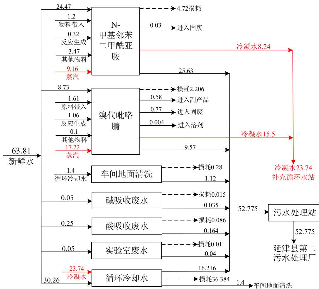
图 3.3-1 本次工程水平衡图 单位: \text{m}^3/\text{d}
