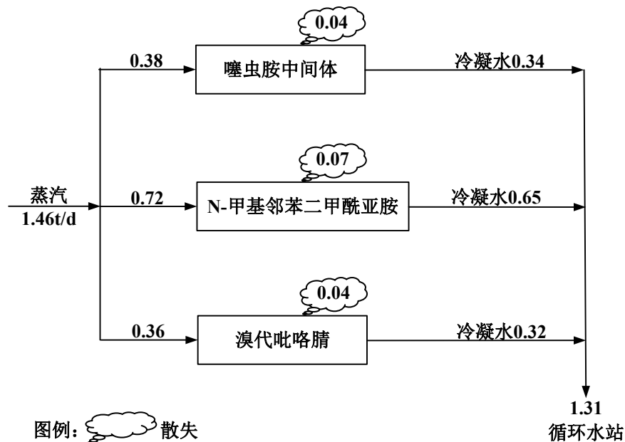
图 3.3-4 全厂蒸汽/凝水平衡图 单位：t/h
