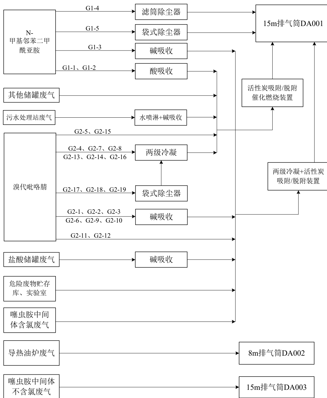
图 3.5-4 全厂废气走向及治理措施示意图
