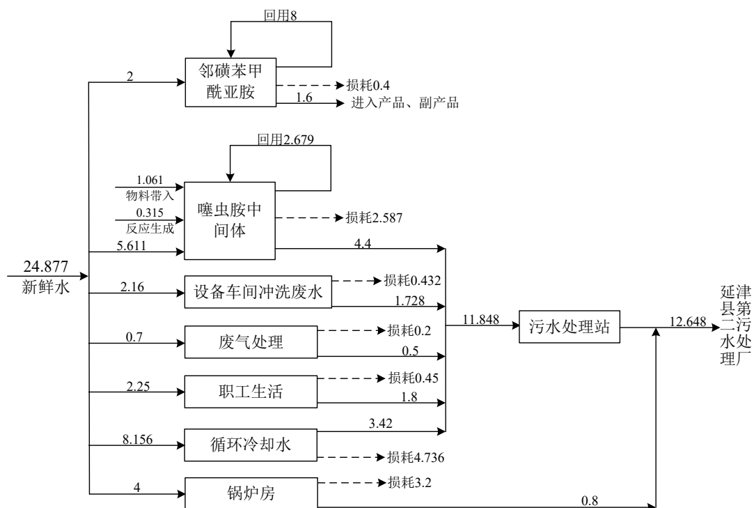
图 3.2-1 现有工程水平衡示意图 单位: \text{m}^3/\text{d}
