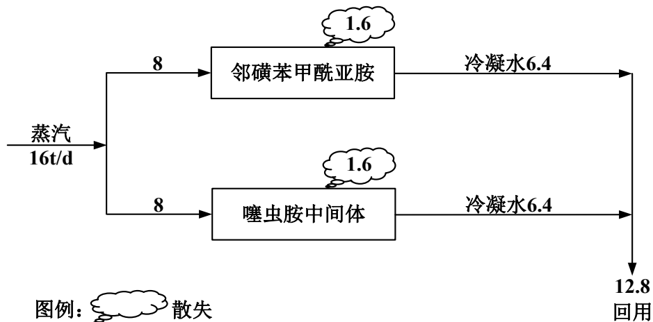
图 3.2-2 现有工程蒸汽平衡示意图 单位: \text{t}/\text{d}
