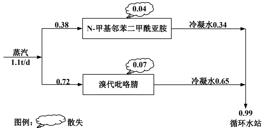
图 3.3-3 本次工程蒸汽/凝水平衡图 单位：t/h
