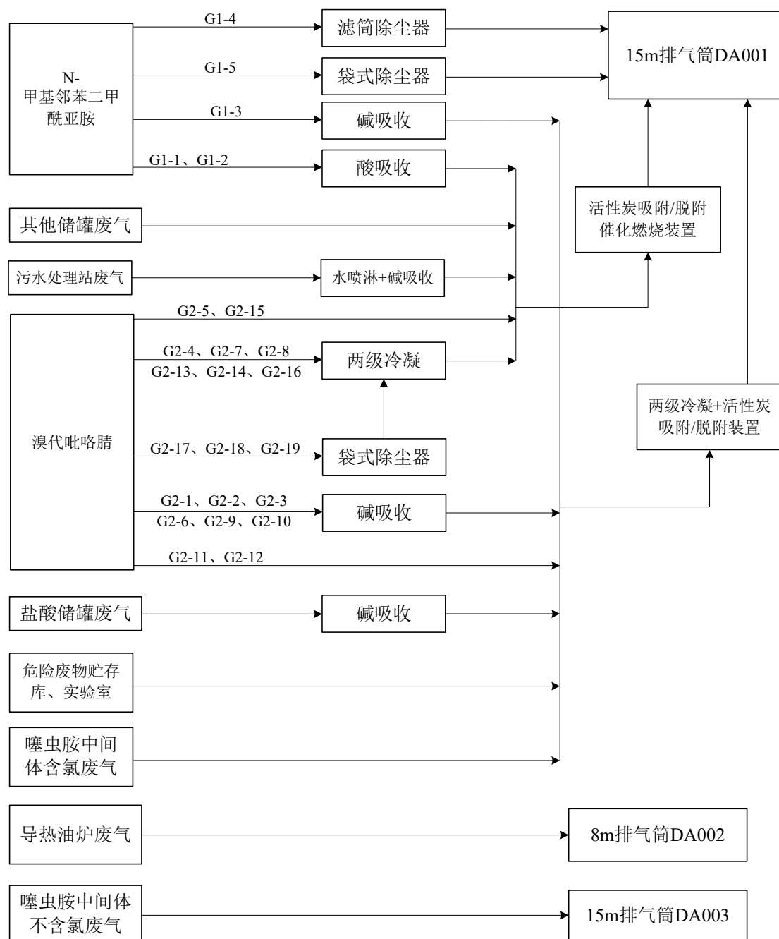
图 7.2-2 全厂废气治理措施示意图
