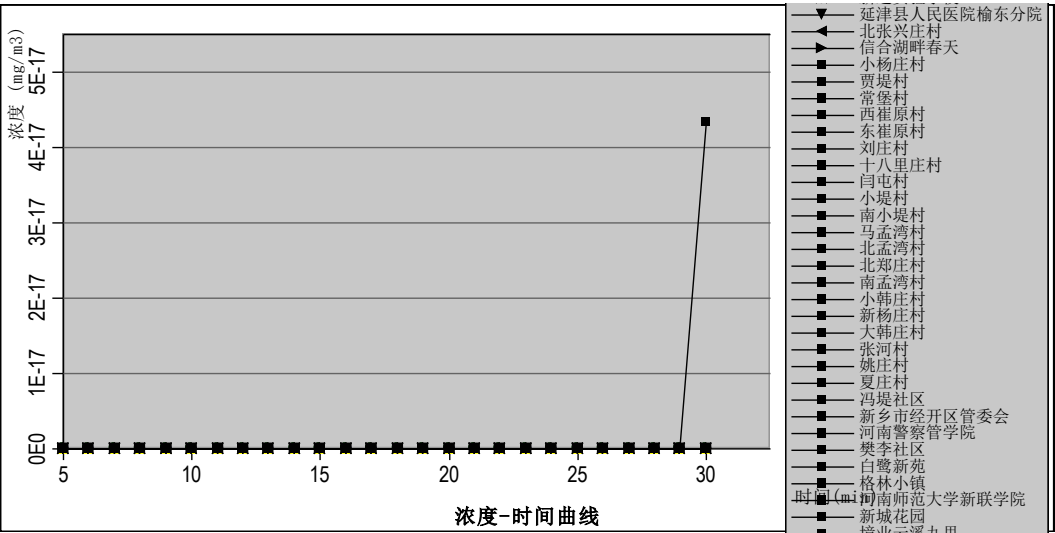
图 6.2-28 最不利气象敏感点 CO 浓度-时间曲线
