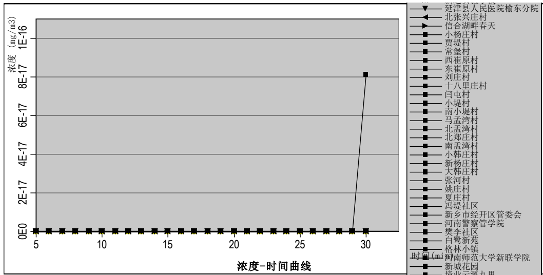
图 6.2-18 最不利气象敏感点甲苯浓度-时间曲线
