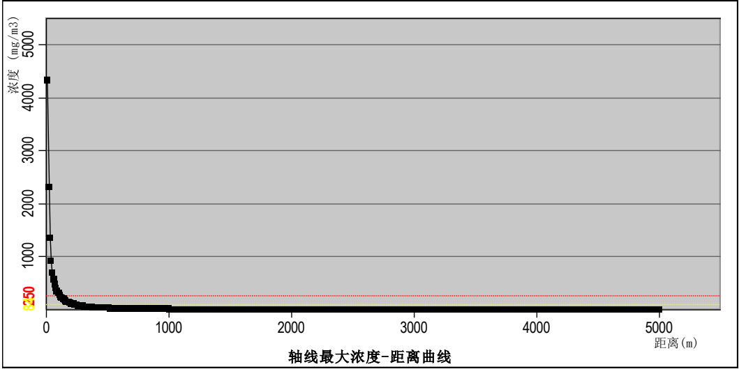
图 6.2-6 最不利气象下风向乙腈最大浓度-距离曲线
