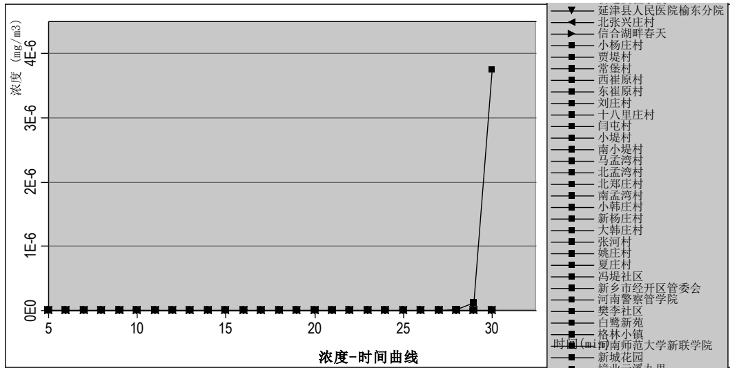
图 6.2-17 最不利气象敏感点氯化氢浓度-时间曲线
