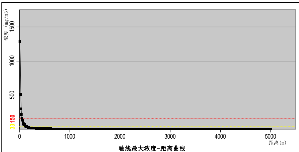
图 6.2-9 最不利气象下风向氯化氢最大浓度-距离曲线
