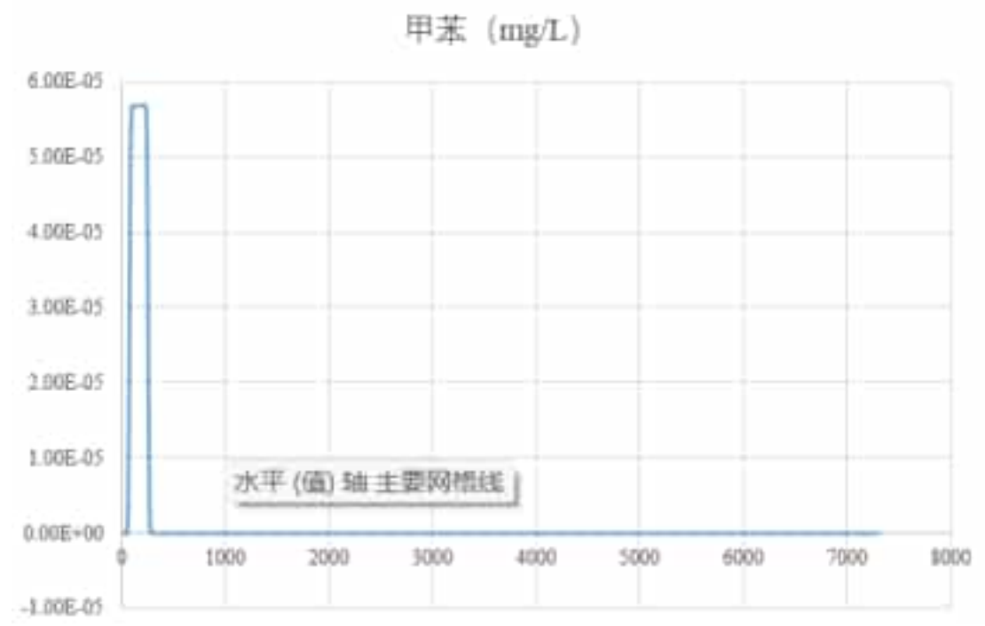
图 5.6-34 厂区下游边界地下水甲苯污染趋势图
