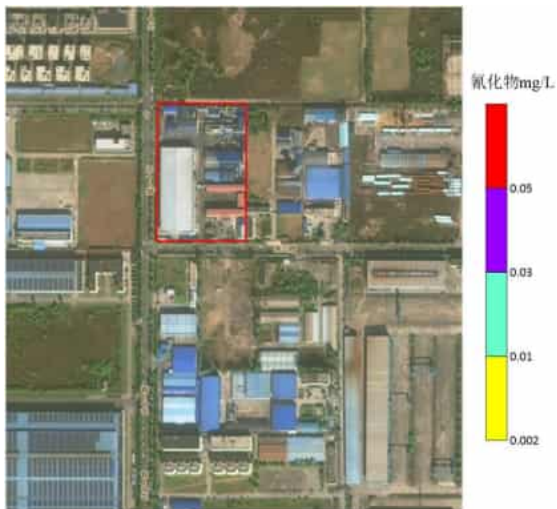
图 5.6-23 100 天污染晕运移分布图
