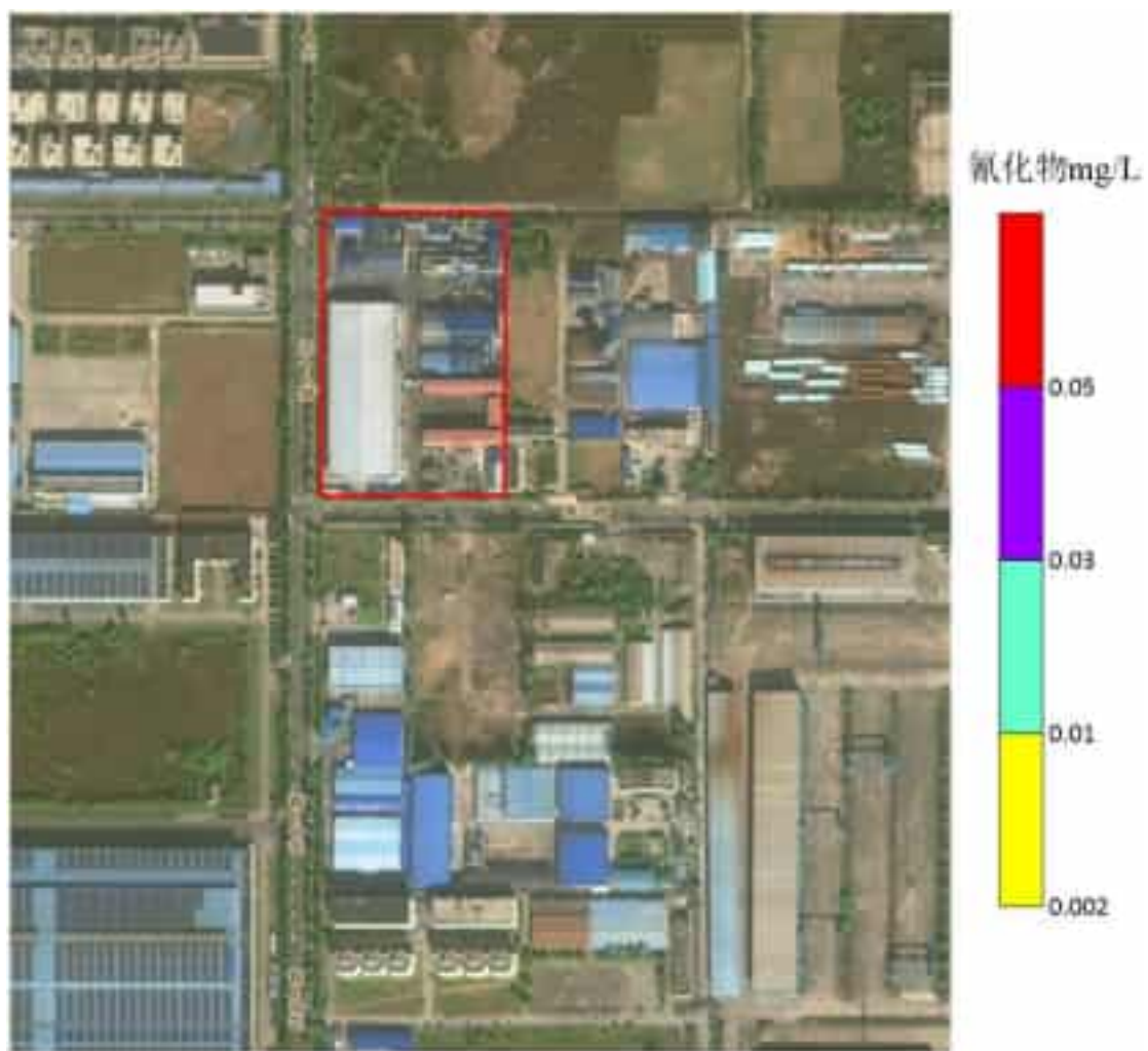
图 5.6-24 1000 天污染晕运移分布图
