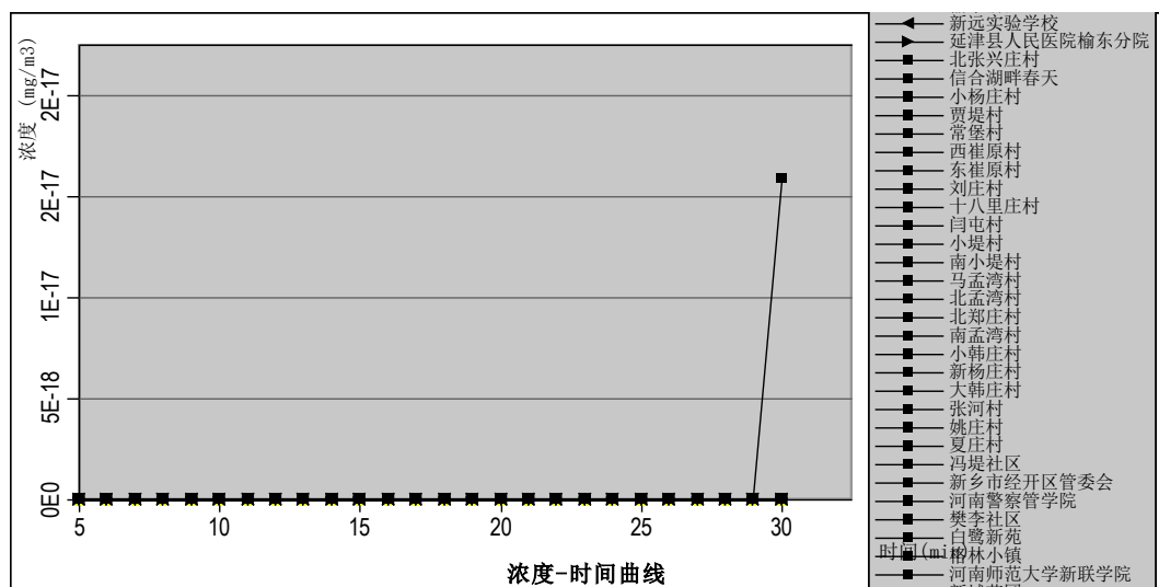
图 6.2-16 最不利气象敏感点溴化氢浓度-时间曲线
