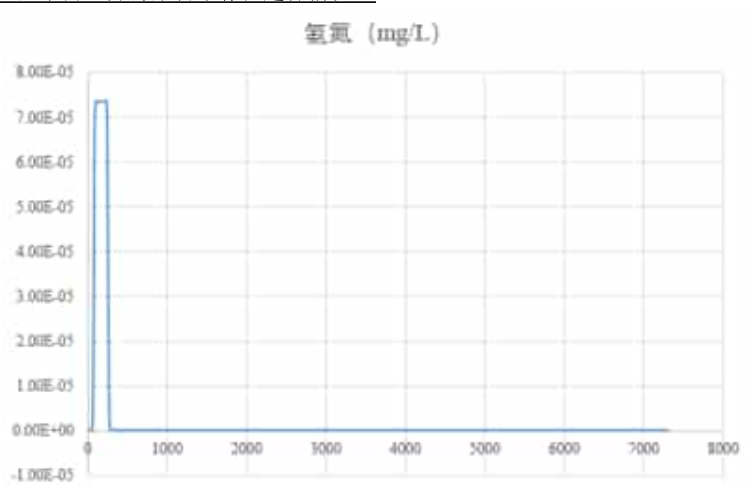
图 5.6-32 厂区下游边界地下水氨氮污染趋势图
