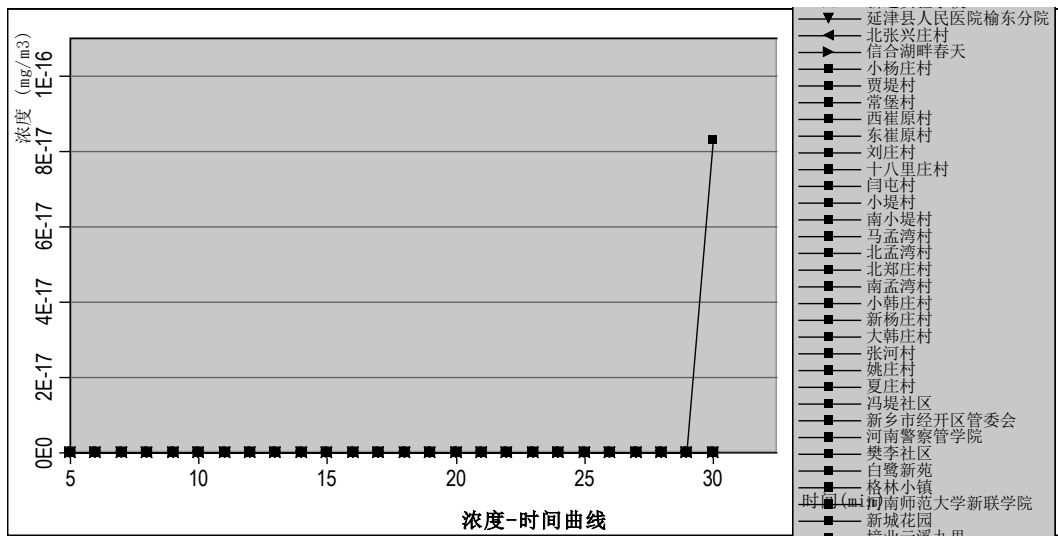
图 6.2-19 最不利气象敏感点甲醇浓度-时间曲线
