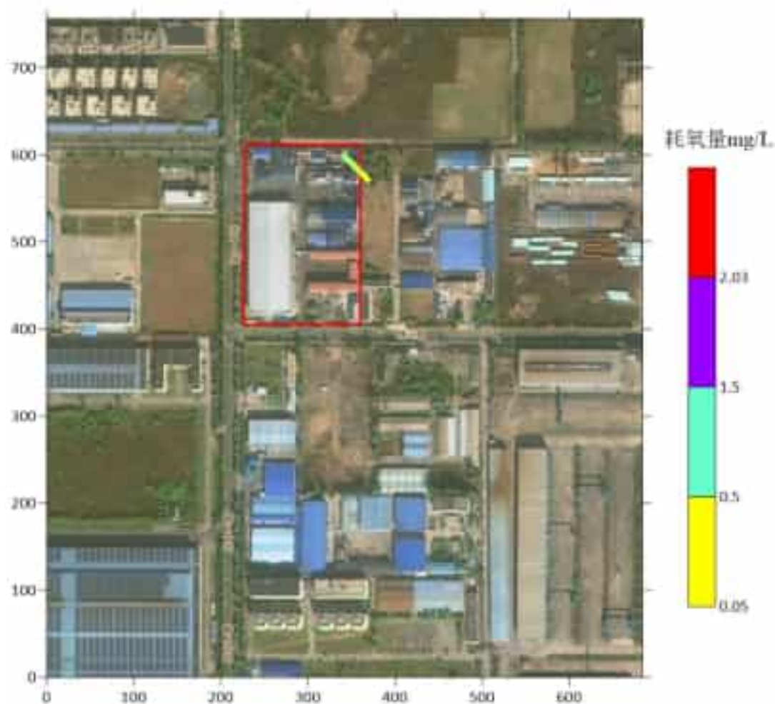
图 5.6-15 100 天污染晕运移分布图
