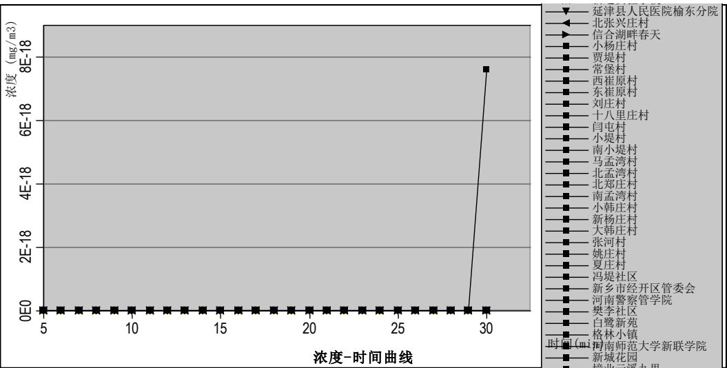
图 6.2-13 最不利气象敏感点 DMF 浓度-时间曲线
