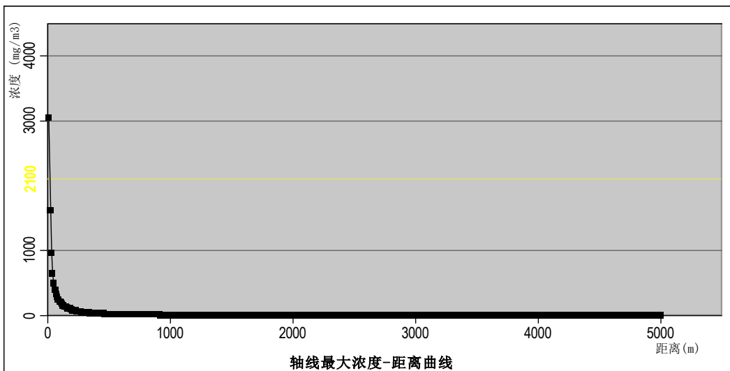
图 6.2-10 最不利气象下风向甲苯最大浓度-距离曲线
