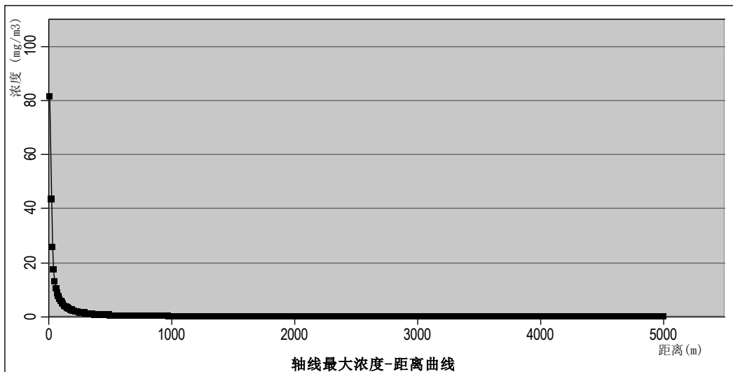
图 6.2-8 最不利气象下风向溴化氢最大浓度-距离曲线
