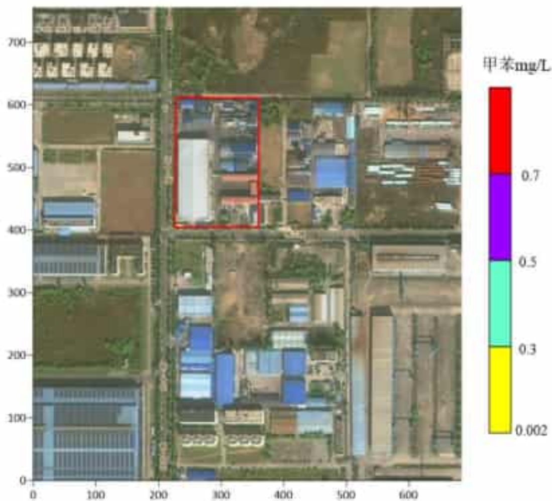
图 5.6-28 1000 天污染晕运移分布图
