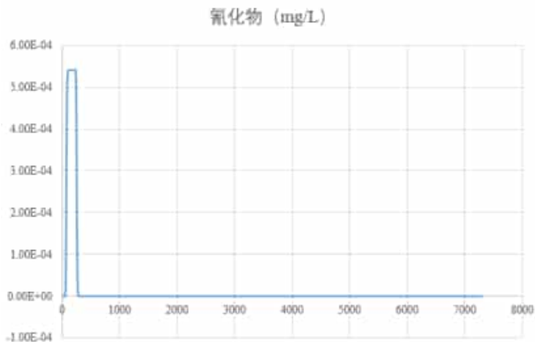
图 5.6-33 厂区下游边界地下水氰化物污染趋势图
