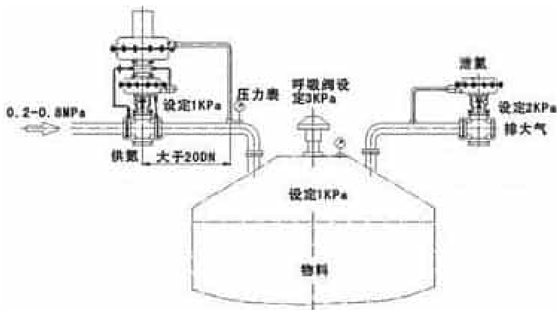
图 3.5-3 罐区氮封装置示意图
