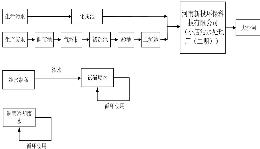
图 6 本次验收项目废水治理工艺路线图
