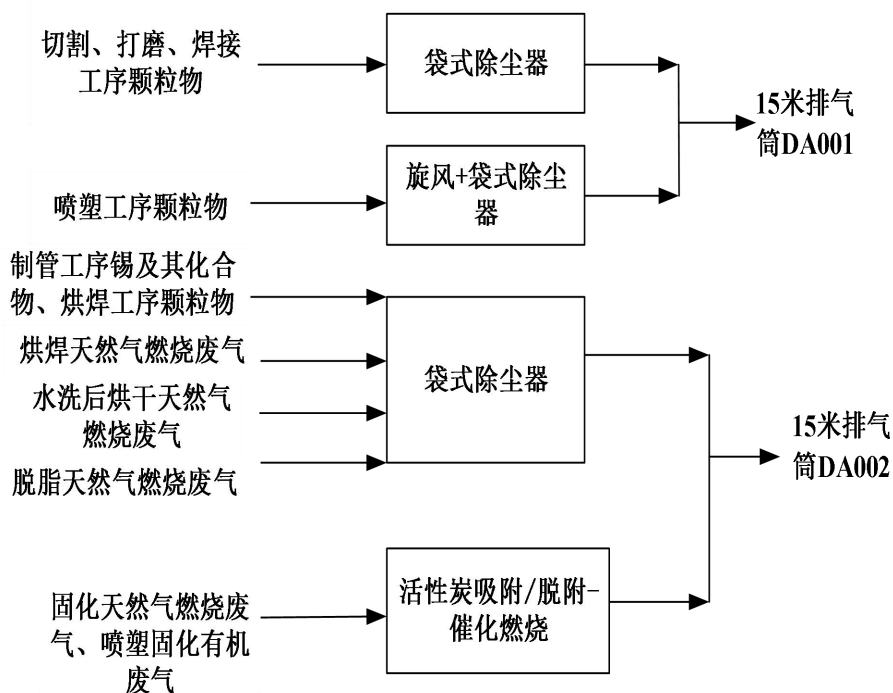
图 5 本次验收项目废气治理工艺路线图
