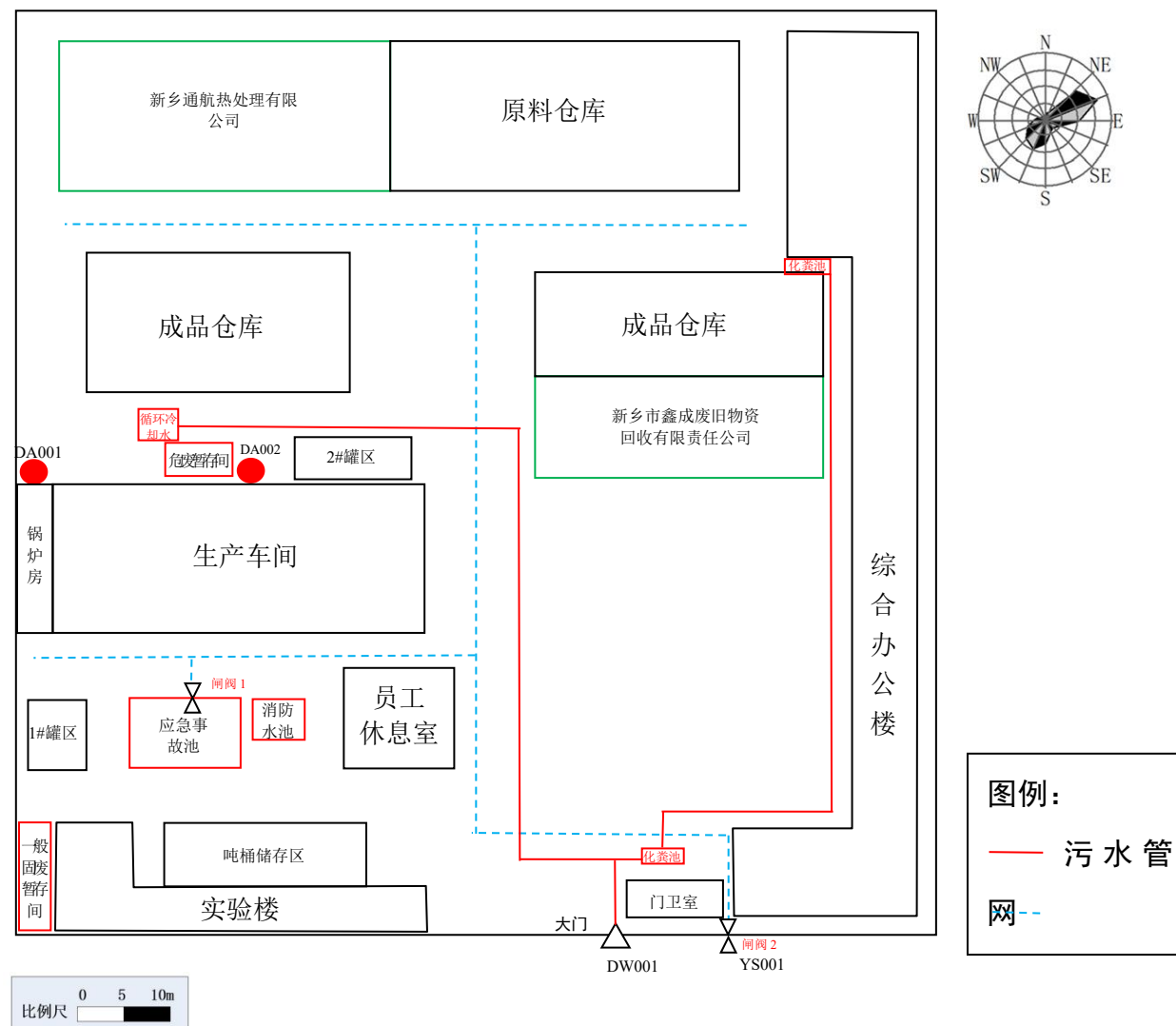
附图 13 项目厂区雨水、污水管网系统及初期雨水、事故废水流向图
