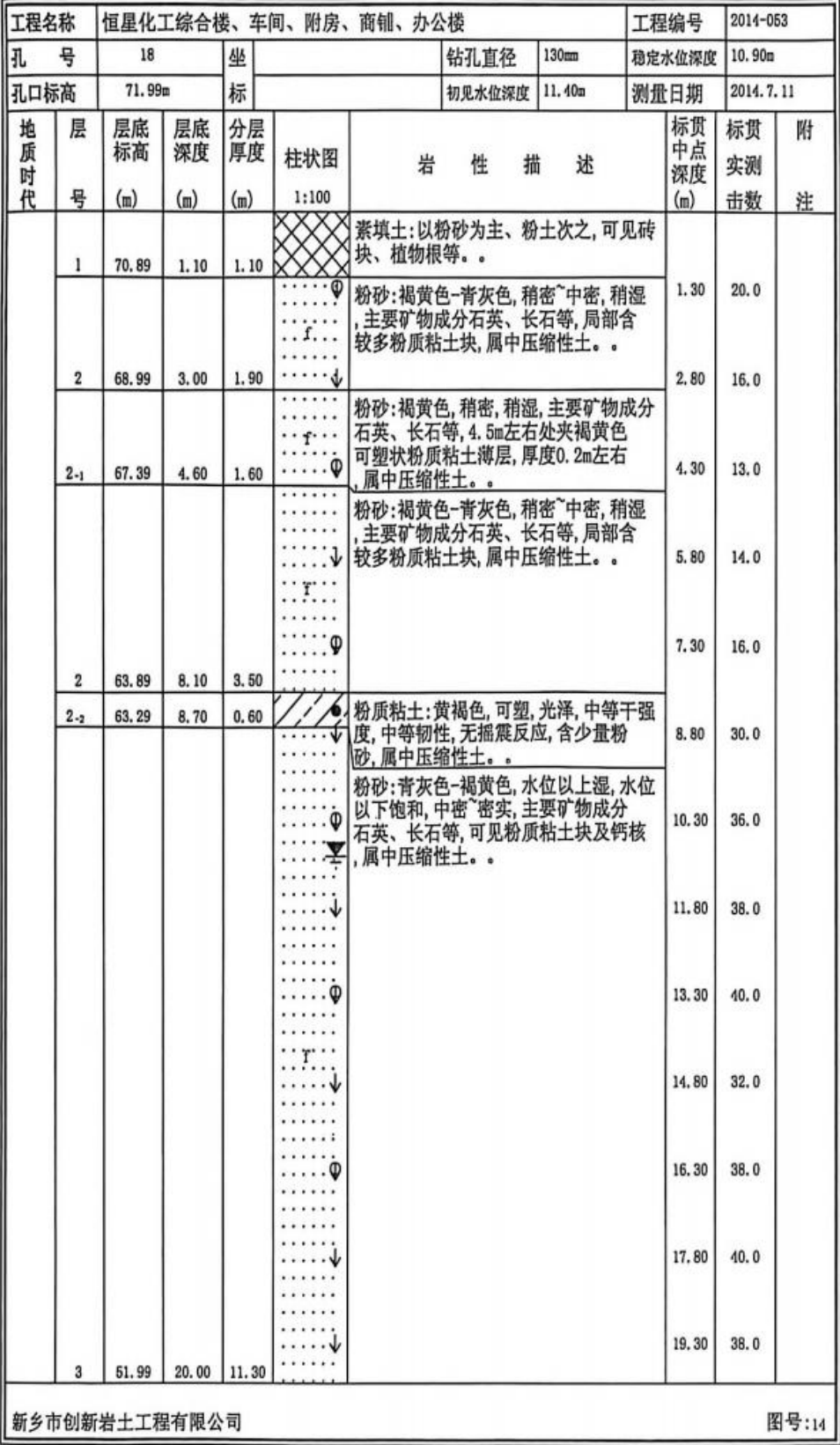
钻 孔 柱 状 图
