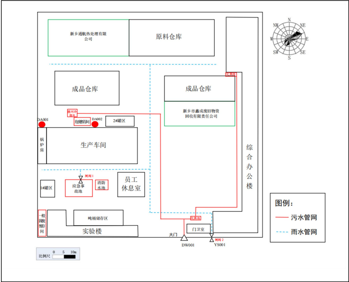
图 5.8-1 项目厂区雨水、污水管网系统及初期雨水、事故废水流向图
