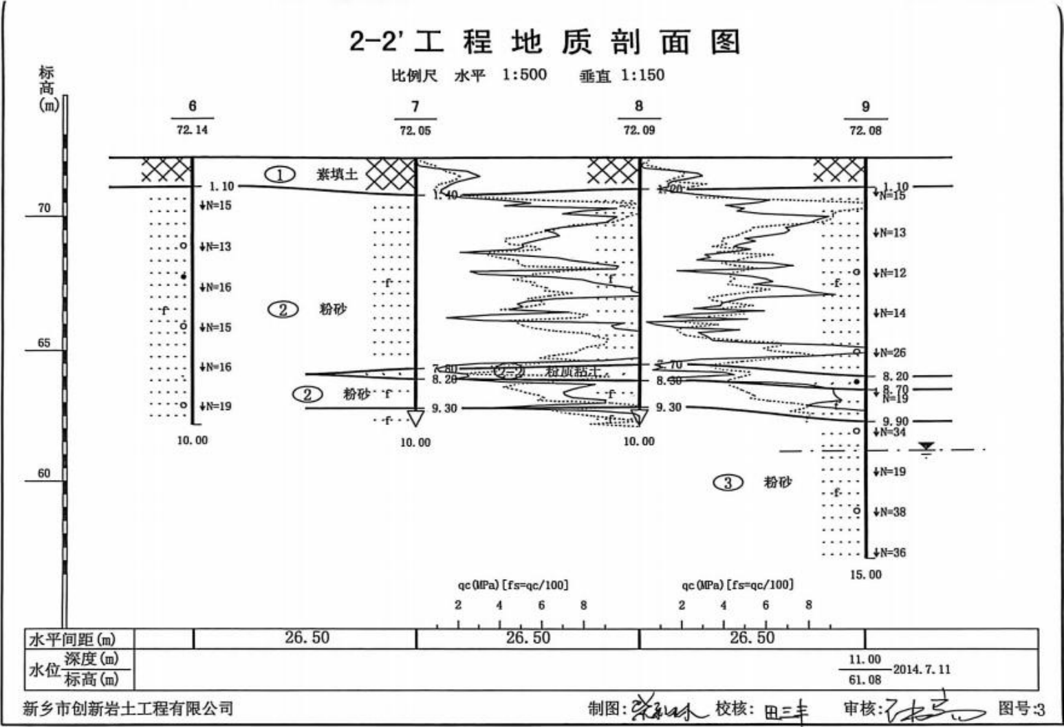
图 5.4-2 厂址工程地质剖面图
