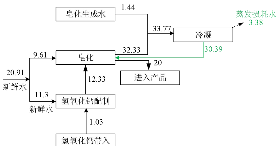
图 3.7-3 本项目水平衡图 单位: kg/t 产品
