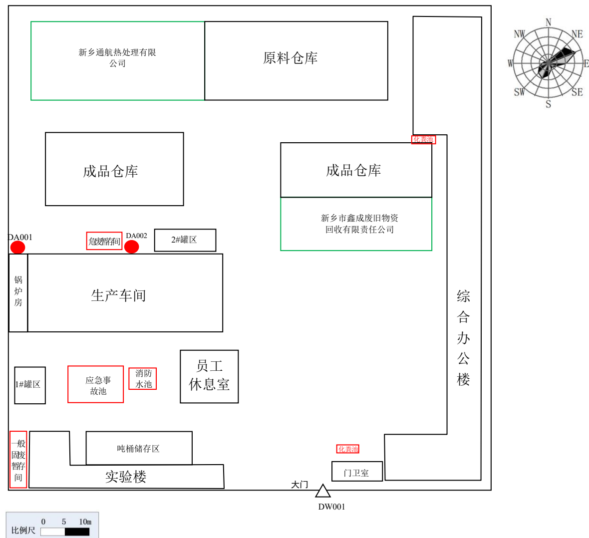
附图2 项目厂区平面图
