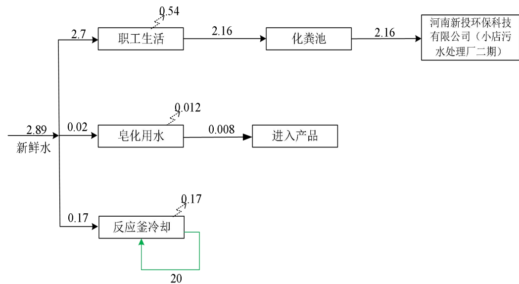
图 3.3-4 现有工程水平衡示意图 单位：m³/d
